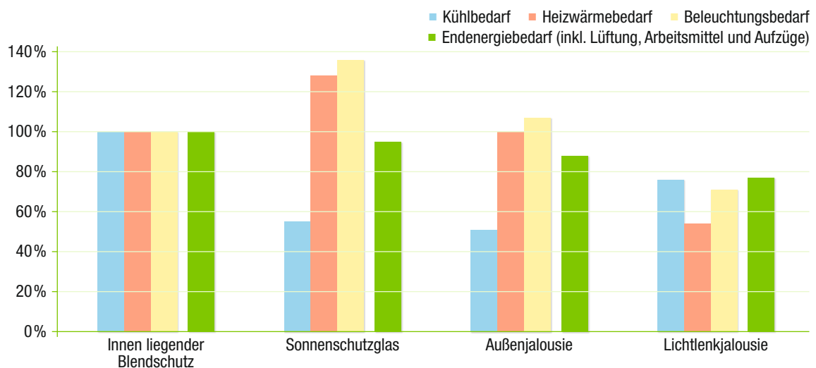
Abb. 7 Auswirkungen der unterschiedlichen Sonnenschutzvarianten auf den Nutz- und Endenergiebedarf im Modellgebäude.
