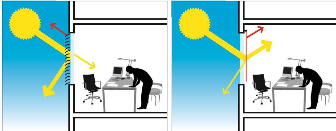
Abb. 3 Funktionsweise von außen und innen liegendem Sonnenschutz. Außen liegender Sonnenschutz verringert den Anteil der Wärmestrahlung, der durch die Fenster in den Raum dringt, durch Absorption und Reflexion. Innen liegender Blendschutz kann diese Funktion nur durch Reflexion ausüben. Die absorbierte Wärme verbleibt im Raum. Um die gegensätzlichen Ansprüche von Sommer und Winter auszugleichen, ist die Kombination beider Systeme zu empfehlen.
